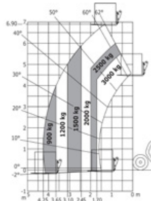
Lastdiagramm Gelände (EN 1459 B)
