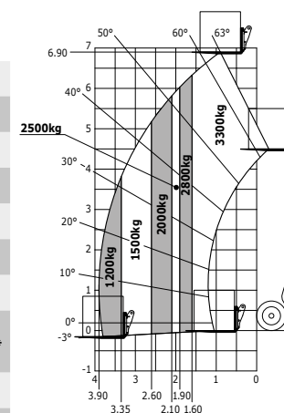
MLT 733-115 / LSU
