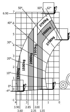
Lastdiagramm Gelände (EN 1459 B)
