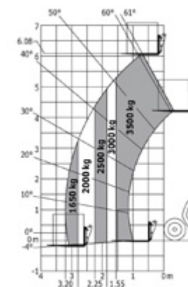
Lastdiagramm Gelände (EN 1459 B)
