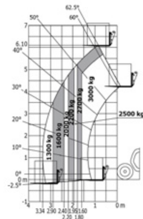
Lastdiagramm Gelände (EN 1459 B)
