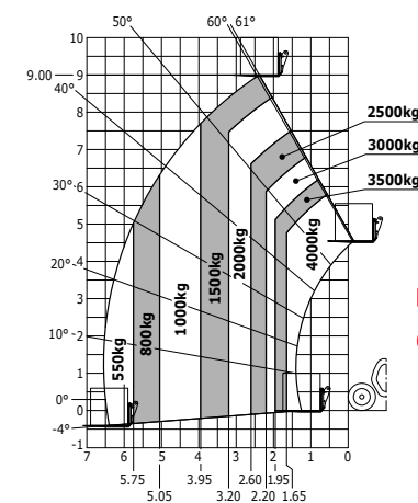
Lastdiagramm Gelände (EN 1459 B)
