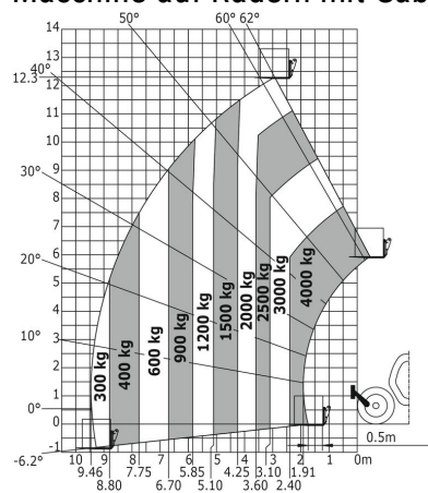
Maschine auf Rädern mit Gabelzinken - mit Niveausgleich
